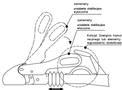
Rys. 5: włączanie urządzenia stabilizującego
