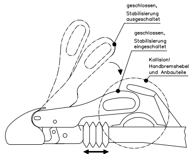
Bild 5: Stabilisierung einschalten
