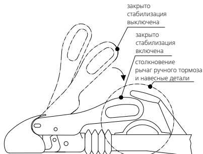
Рисунок 5: Включить стабилизацию
