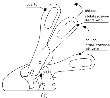
Figura 6: attivazione della stabilizzazione disaccoppiamento
