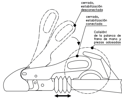
Figura 5: Activar estabilización
