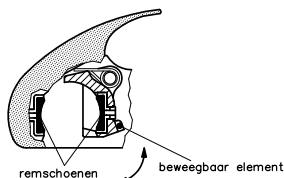
Afbeelding 9: plaatsing van de frictie-elementen
