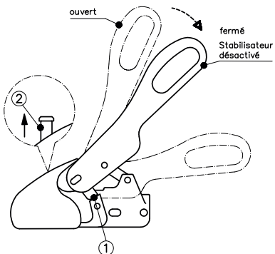
Croquis 4 : Accrochage
