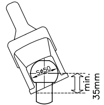
Kuva 1: Vetoauton vetokoulu
