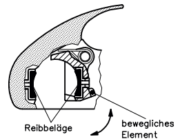
Bild 9: Anordnung der Reibelemente
