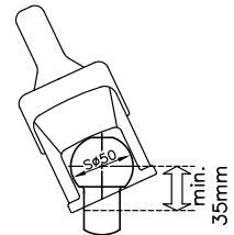
Figura 1: asta sferica del veicolo trainante
