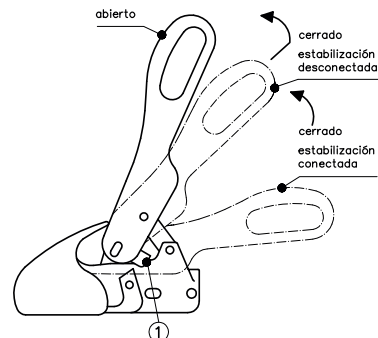
Figura 6: Desactivar estabilización Desacoplar
