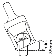
Billede 1: Kuglestang trækøretøj
