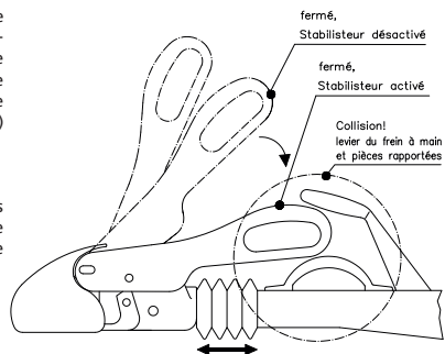
Croquis 5 : Activation de la stabilisation
