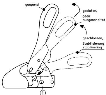
Afbeelding 6: stabilisator uitschakelen loskoppelen
