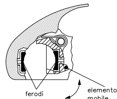
Figura 9: disposizione degli elementi di frizione
