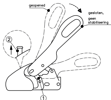
Afbeelding 4: aankoppeling
