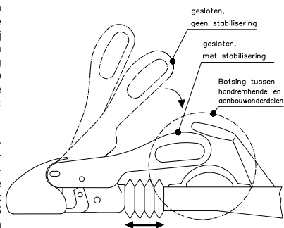
Afbeelding 5: stabilisator inschakelen
