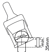
Figura 1: Barra de esfera Vehículo tractor
