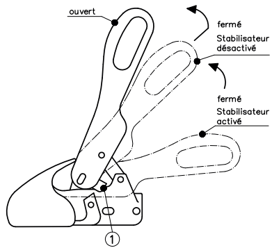
Croquis 6 : Désactivation de la stabilisation Décrochage
