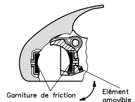
Croquis 9 : Agencement des éléments de friction
